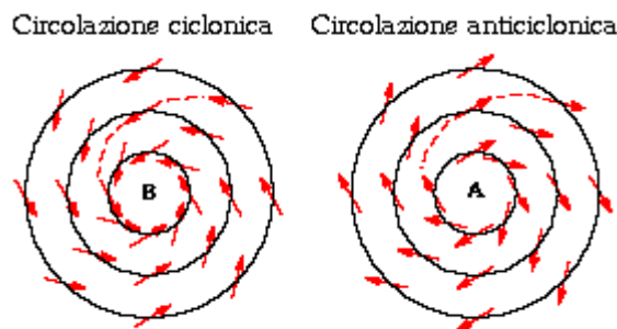
Grafico 2 - Andamento dei venti nell'emisfero nord
