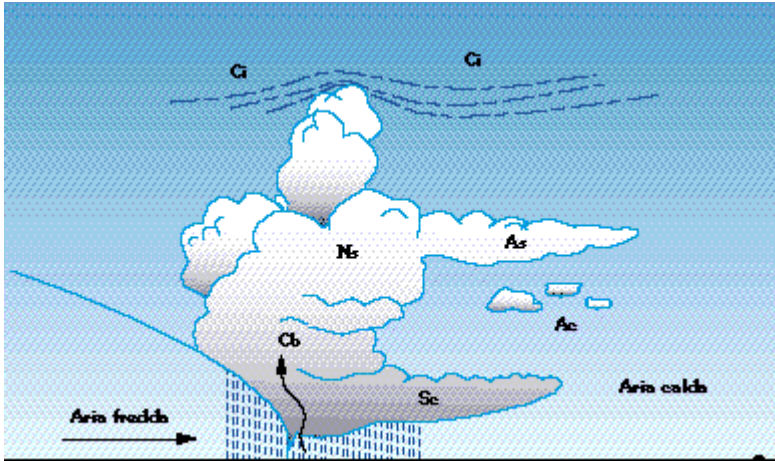
Grafico 4 - Fronte freddo con le sue nubi caratteristiche
