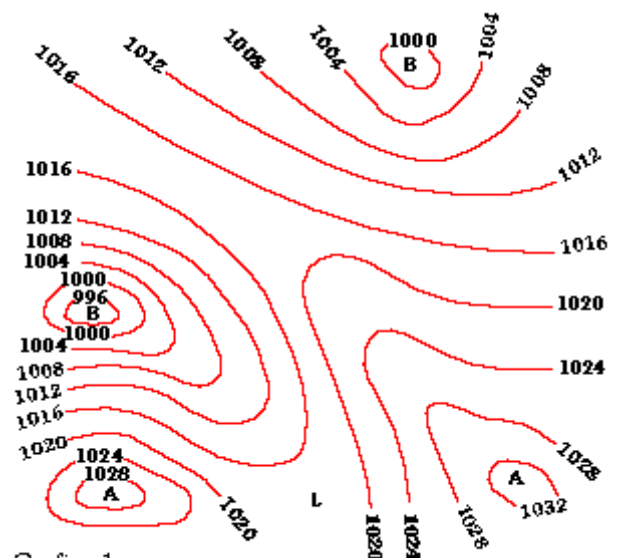
Grafico 1 A=Anticiclone B=Depressione L=Pressione livellata
