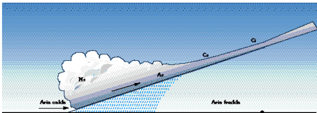
Grafico 3 - Il fronte caldo con le sue nubi caratteristiche
